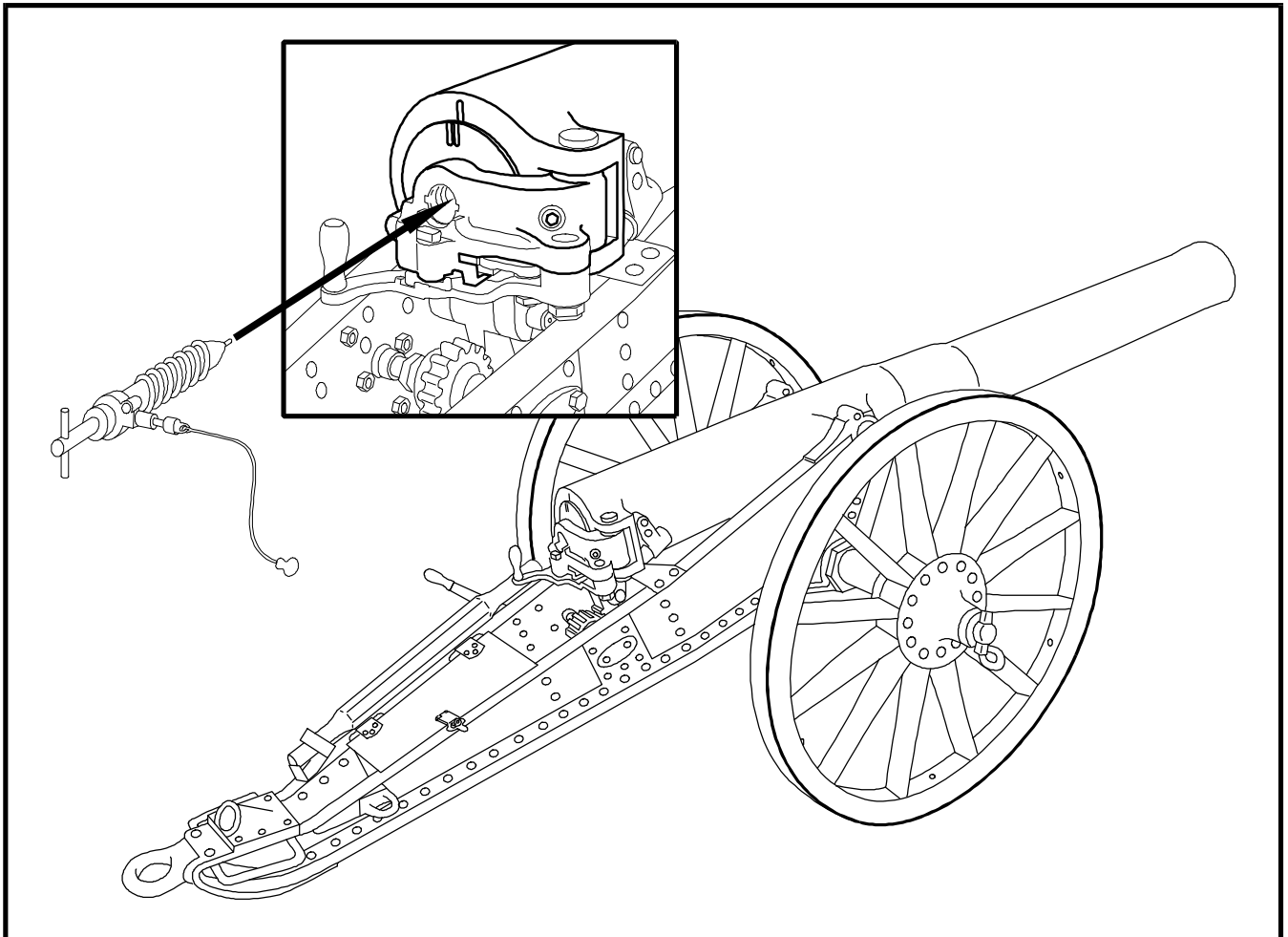
Figure 4-1 Naval field gun Figure 4-1 Pièce d'artillerie navale de campagne
